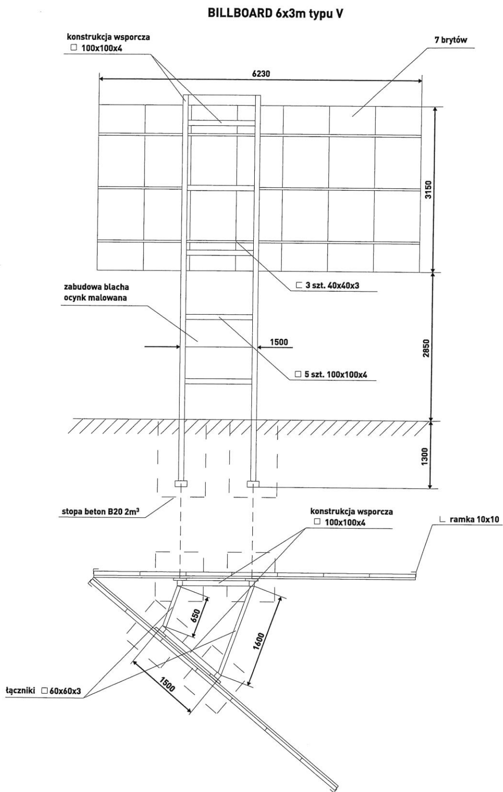
Rys. 1 – projekt istniejącej tablicy informacyjnej w kształcie litery V
